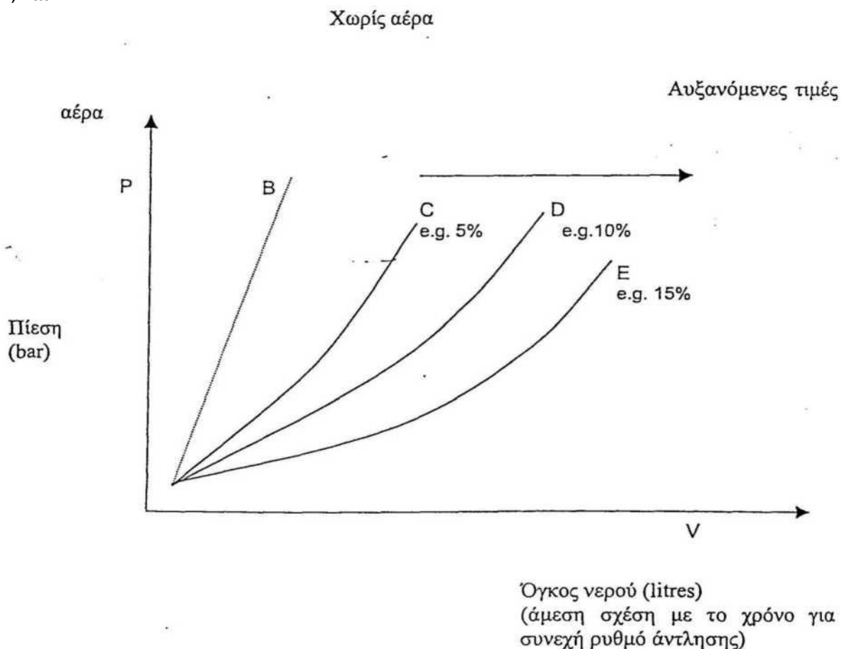
Σχήμα 4 : Σχέση πίεσης / όγκου κατά την διάρκεια της δοκιμής πίεσης.
