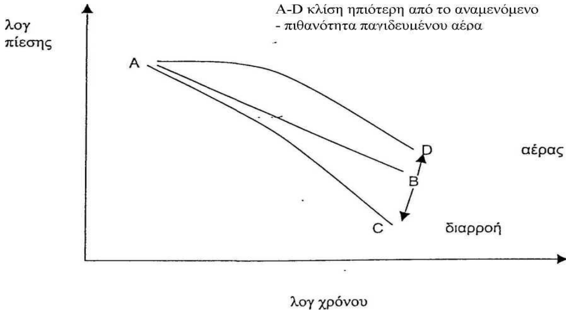
Σχήμα 3 : Διάγραμμα λογαρίθμου πίεσης συναρτήσει του λογαρίθμου του χρόνου.
